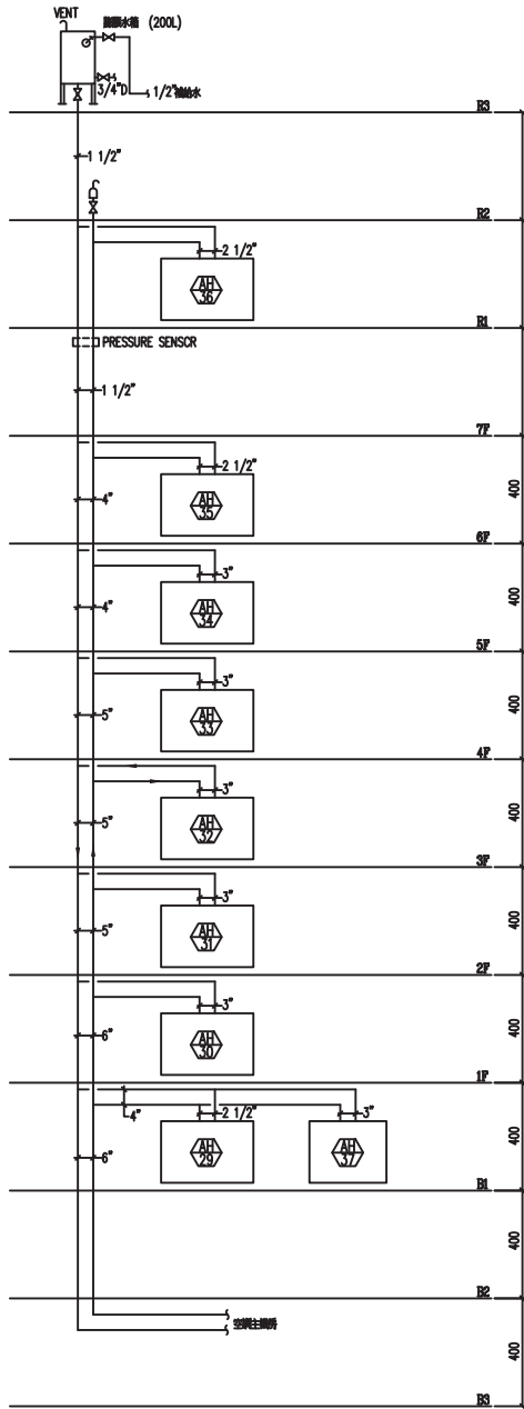
C區冰水管昇位圖
