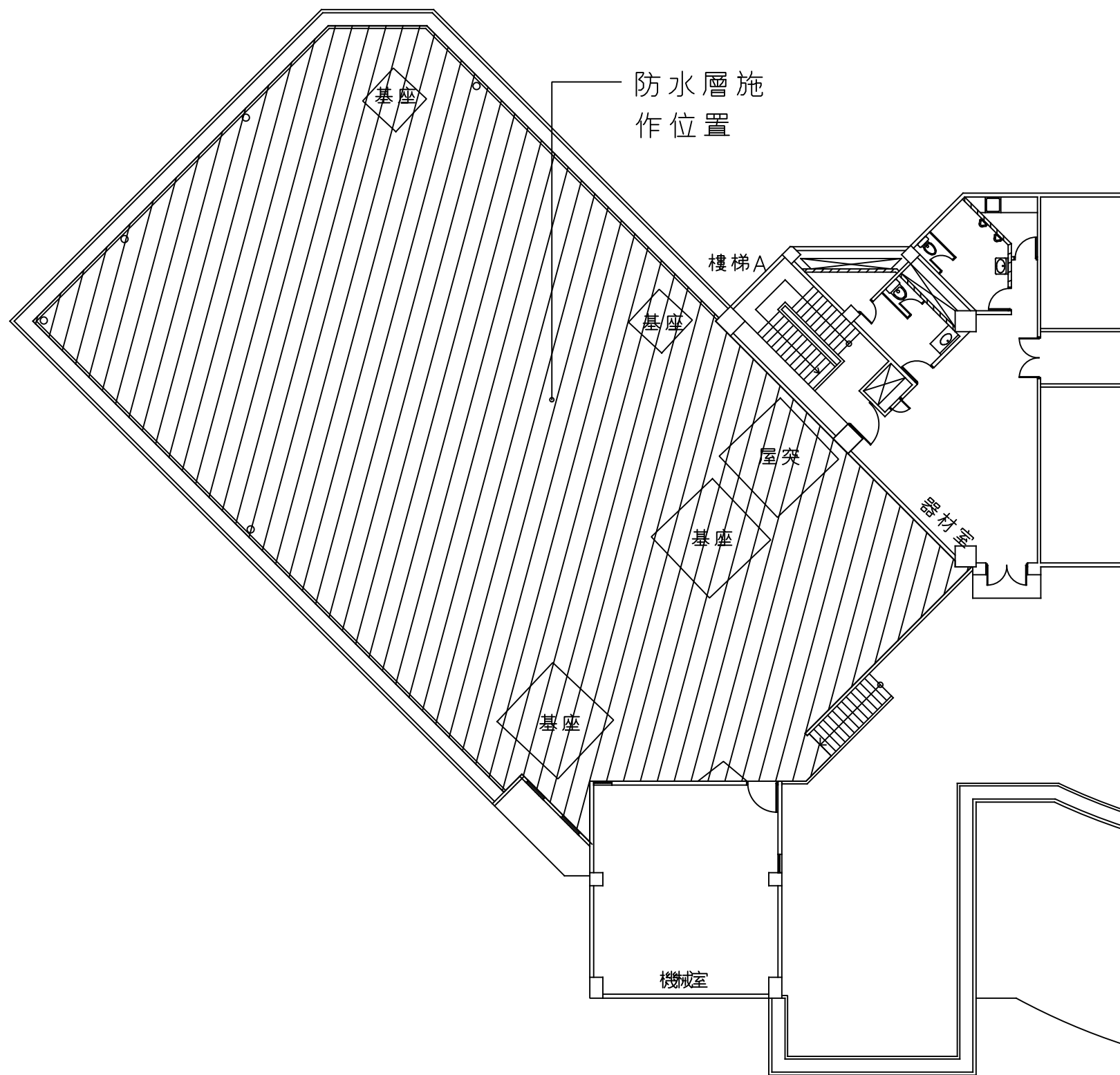
八層施工位平面圖 S:1/200
