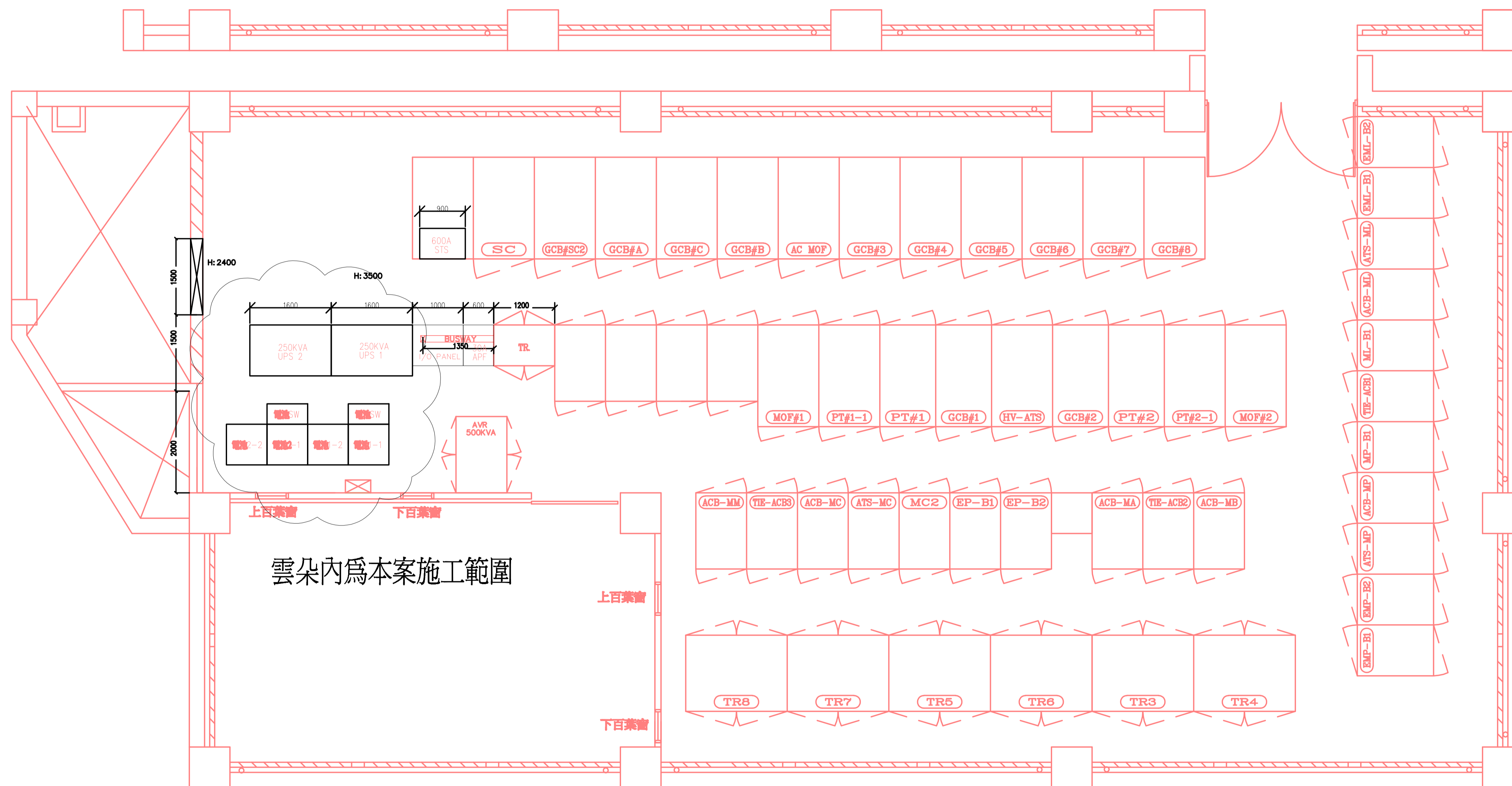
B 棟重電室 UPS 開關盤平面圖
