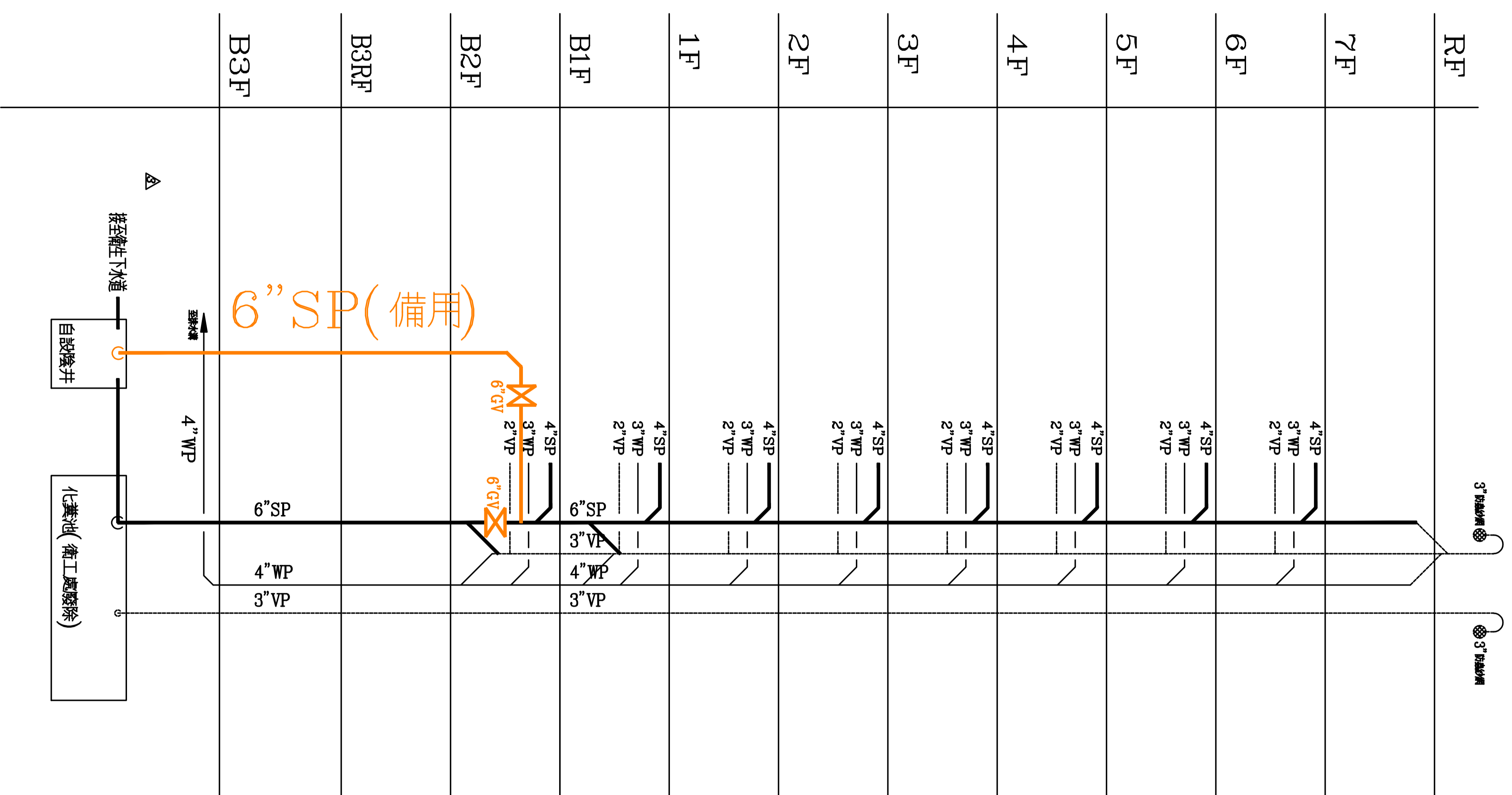
C棟污水昇位圖
